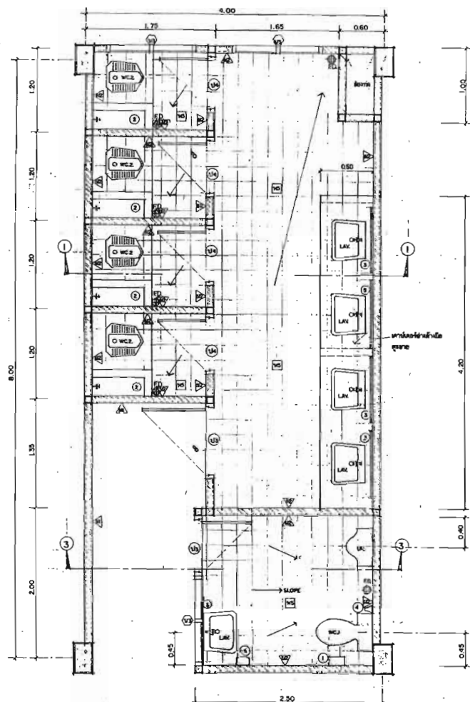
แบบขยายห้องน้ำ - ล้วม ผู้หญิง (ชั้นล่าง)
