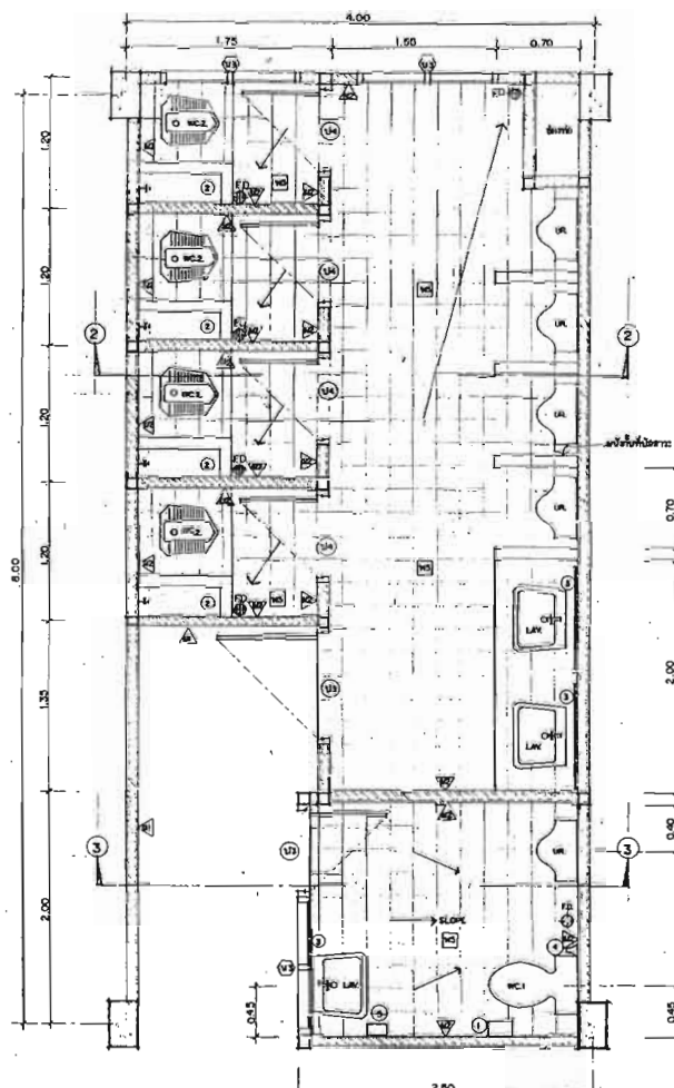
แบบขยายห้องน้ำ - ล้วน ผ้ายาย (ชั้นฉาบ)
