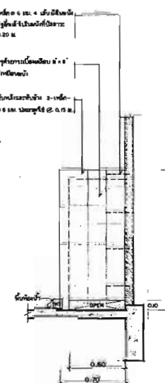
ขยายผนังกันที่ปลาดาว
