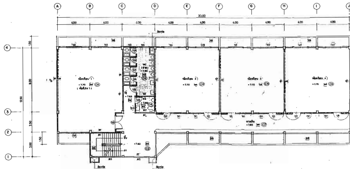
แปลนพื้นชั้นล่าง มาตรา ๘๖
