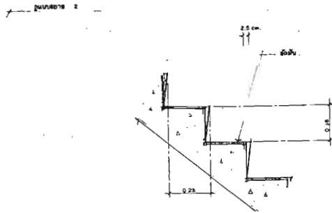
แบบขยาย ขนาดจริง 1:10
