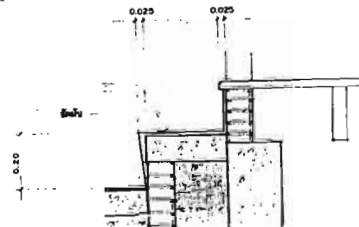
แบบขยาย 5 ขนาดจริง 1:10
