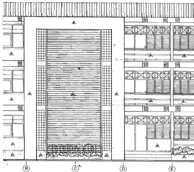
รูปด้านหน้าอาคาร มาตราส่วน 1:50
